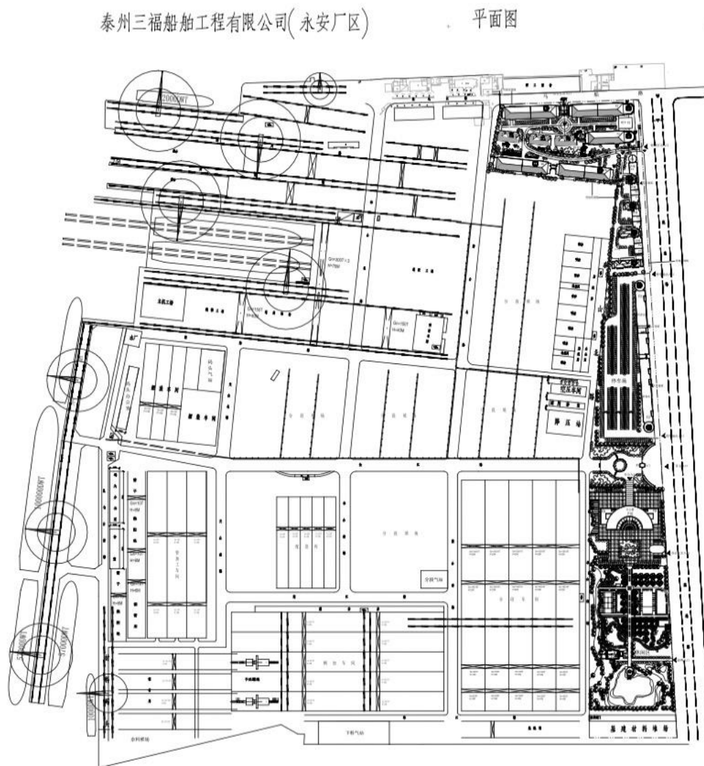
图 3-4 平面布局图
