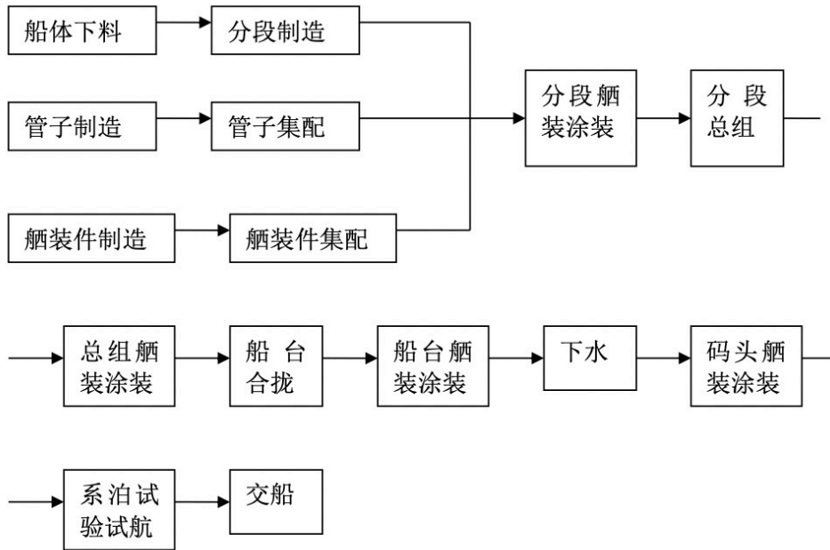
图 3-3 生产工艺流程
